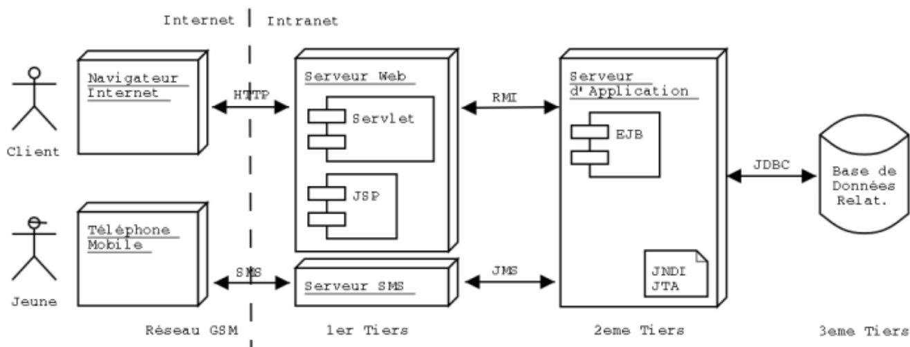
Architecture d'une application distribuée typique
